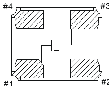
内部链接 < 顶视图 > Internal Connections < Top View >
